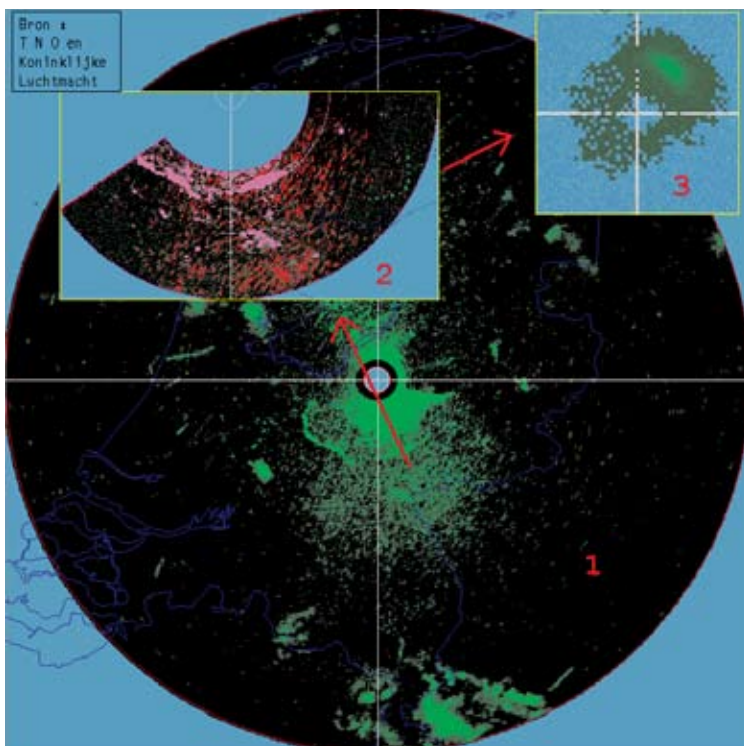
Figuur 2.2. Visualisatie van de werking van het ROBIN systeem. (1) Het “ruwe” radarbeeld waarop “ground clutter” (reflectie van objecten op de grond), regen, vliegtuigen en vogels te zien zijn. (2) Het met ROBIN bewerkte ruwe beeld, waarop nu in rood de “tracks” van de vogels zijn aangegeven. (3) Een vector plot van de vliegrichting van de vogels. Overgenomen van de website van TNO: www.tno.nl .
